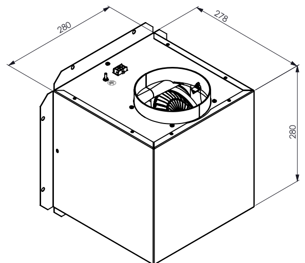
Box motore / Box engine
